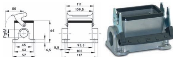
EPIC® H-B 16 SGRL-LB Gehäusebauform H-B. Der Industriestandard.
