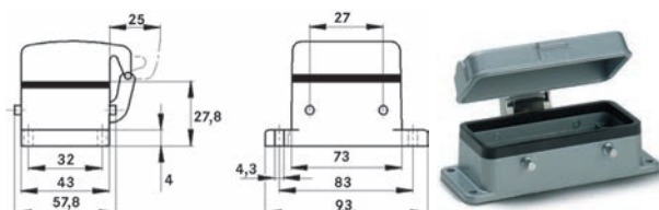
EPIC® H-B 10 AD-BO Gehäusebauform H-B. Der Industriestandard.
