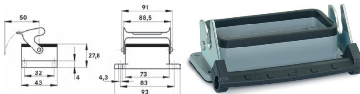
EPIC® H-B 10 AD-LB Gehäusebauform H-B. Der Industriestandard.
