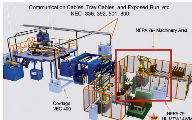
Das Schema einer industriellen Maschine zeigt wesentliche Anwendungen von Kabeln und Leitungen mit Verweis auf die zugehörigen Abschnitte in NEC®/NFPA. ‚NEC®‘ ist ein Markenzeichen der National Fire Protection Association <NFPA>.
