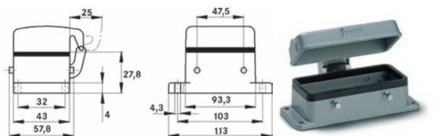
EPIC® H-B 16 SGR-LB Gehäusebauform H-B. Der Industriestandard.
