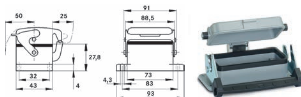
EPIC® H-B 10 AG Gehäusebauform H-B. Der Industriestandard.
