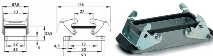
EPIC® H-B 10 AD-BO Gehäusebauform H-B. Der Industriestandard.
