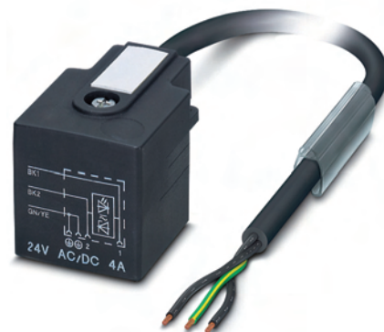
S/A-Kabel: 3-polig, Ventilstecker auf freies Leitungsende
