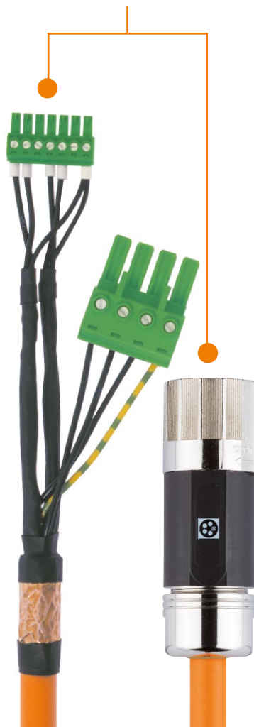
ÖLFLEX® CONNECT SERVO podle standardu INDRAMAT®
