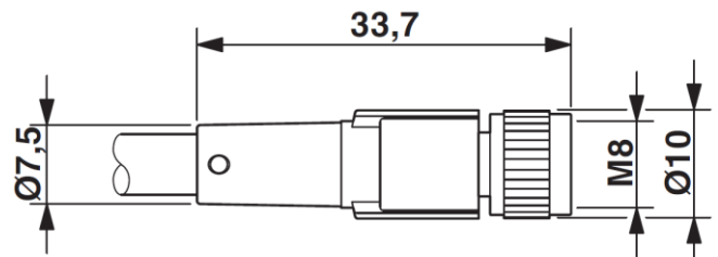
Buchse M8 x 1, gerade
