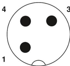
Polbild M12-Stecker, 3-polig, A-kodiert, Ansicht Stiftseite
