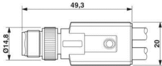
Stecker M12 x 1, Y-Verteiler
