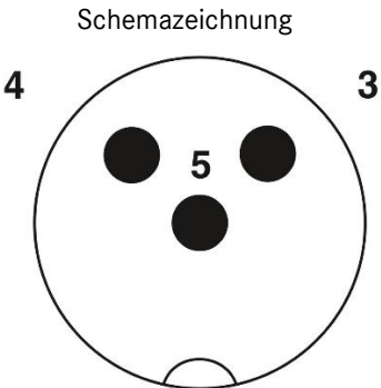
Polbild M12-Stecker, 3-polig, A-kodiert, Ansicht Stiftseite
