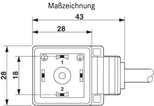
Ventilstecker, Bauform A
