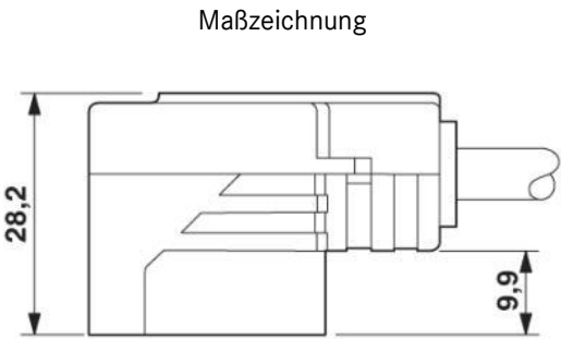
Ventilstecker, Bauform A, Seitenansicht
