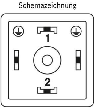
Polbild Ventilstecker, Bauform A
