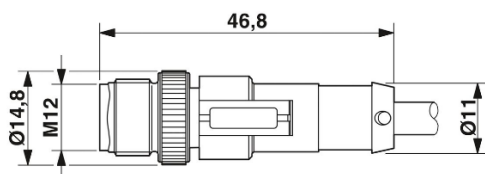
Stecker M12 x 1, gerade, geschirmt, A-kodiert
