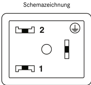
Polbild Ventilstecker, Bauform B
