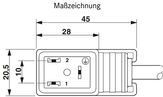
Ventilstecker, Bauform B
