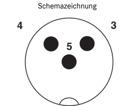
Polbild M12-Stecker, 3-polig, A-kodiert
