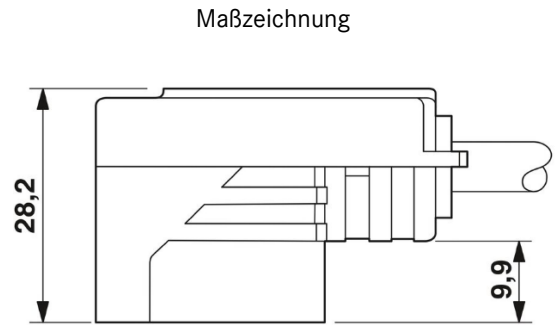
Ventilstecker, Bauform B1, Seitenansicht
