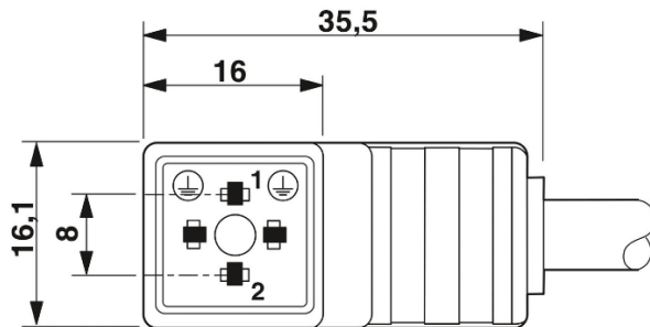
Ventilstecker, Bauform C
