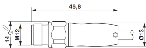
Stecker M12 x 1, gerade, geschirmt
