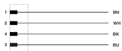
Kontaktbelegung des M12-Steckers und der M12-Buchse
