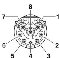
Stecker
