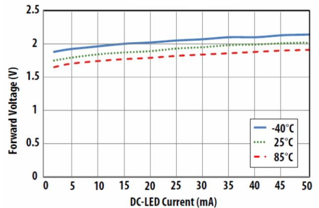
Diagramm Durchlass-Spannung
