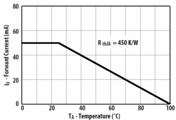
Diagramm Durchlass-Strom
