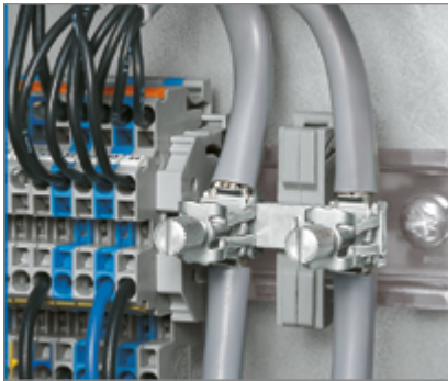
Obejmy zaciskowe do ekranu na szynie równoległej do szyny montażowej z przewodzącą stopką na TS 35 ④ ⑤ ⑥ ⑦ ㉑ ㉒ ㉓
