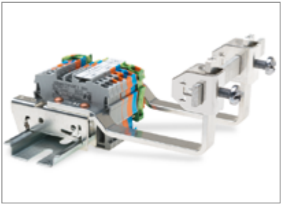
Szyna zbiorcza usytuowana pionowo mocowana na metalowym wsporniku do przesuwanego uchwyty teowego ⑭ ⑮ ⑯ ㉑ ㉒ ㉓ ㉔ ㉕ ㉖ ㉗ ㉘ ㉙
