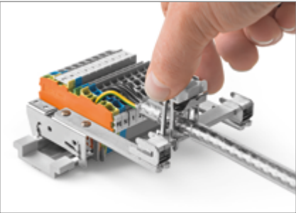
Montaż obejmy zaciskowej do ekranu ze sprężyną na szynie zbiorczej mocowanej na jednostronnych prostych wspornikach metalowych ① ② ③ ⑭ ⑮ ⑯ ⑰ ㉑ ㉒
