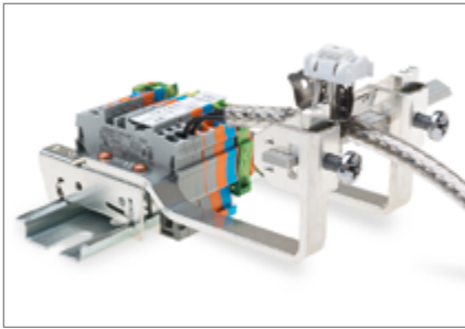
Obejma zaciskowa do ekranu ze sprężyną na szynie zbiorczej usytuowanej poziomo mocowanej na metalowym wsporniku do przesuwanego uchwyty teowego ① ② ③ ⑭ ⑮ ⑯ ㉑ ㉒ ㉓ ㉔ ㉕ ㉖ ㉗ ㉘ ㉙
