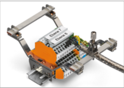
Obejma zaciskowa do ekranu ze śrubą na szynie zbiorczej mocowanej na dwustronnych ukośnych wspornikach metalowych ④ ⑤ ⑥ ⑦ ⑭ ⑮ ⑯ ㉑ ㉒
