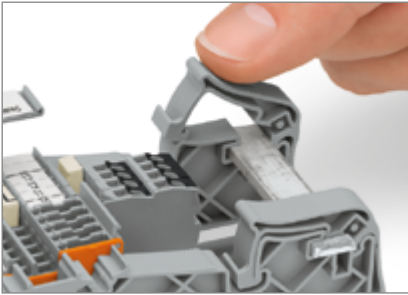
Montaż szyny zbiorczej na izolowanych wspornikach ⑭ ⑮ ⑯ ㉚
