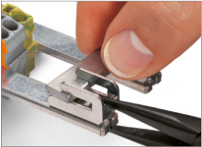
W celu demontażu szyny zbiorczej należy ścisnąć obcęgami sprężynę dociskającą szynę ⑭ ⑮ ⑯ ㉑ ㉒
