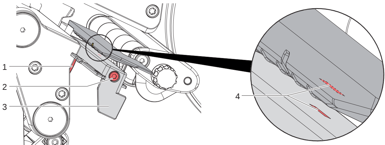
Bild 24 Etikettenlichtschanke reinigen
