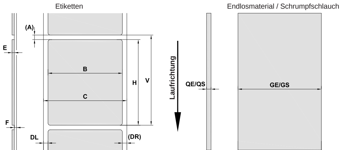
Bild 26 Maße Etiketten / Endlosmaterial
