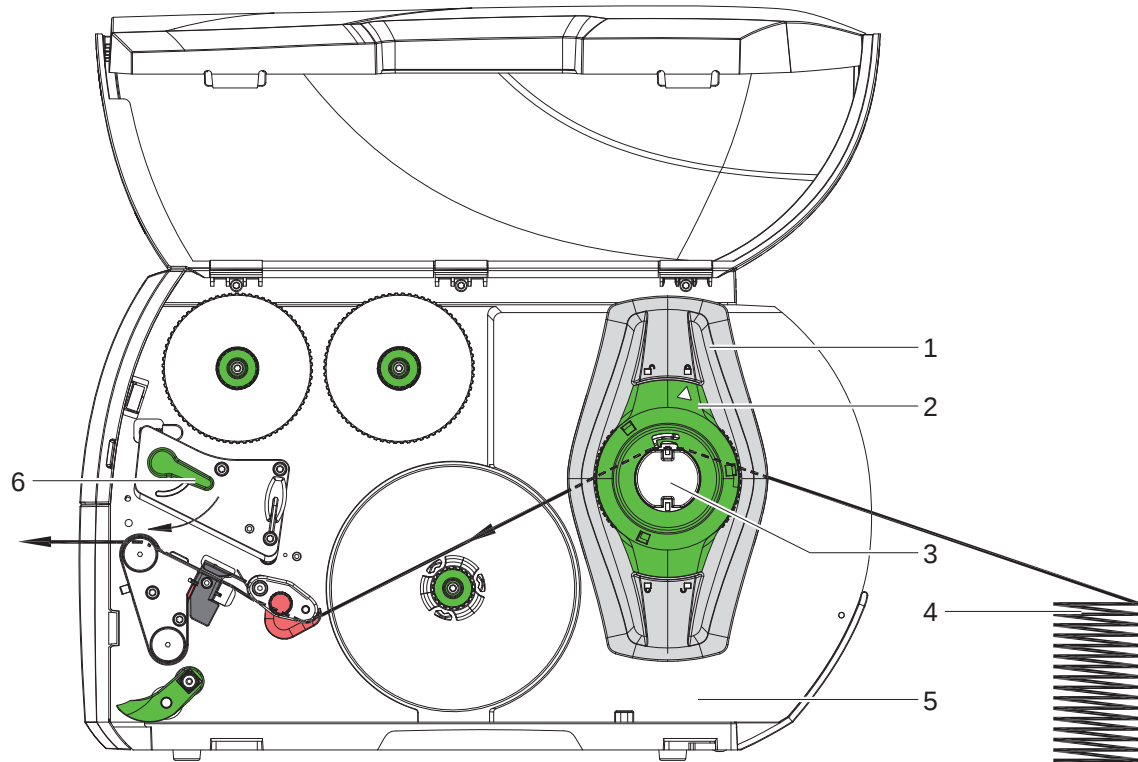
Bild 17 Papierlauf mit Leporello-Etiketten
