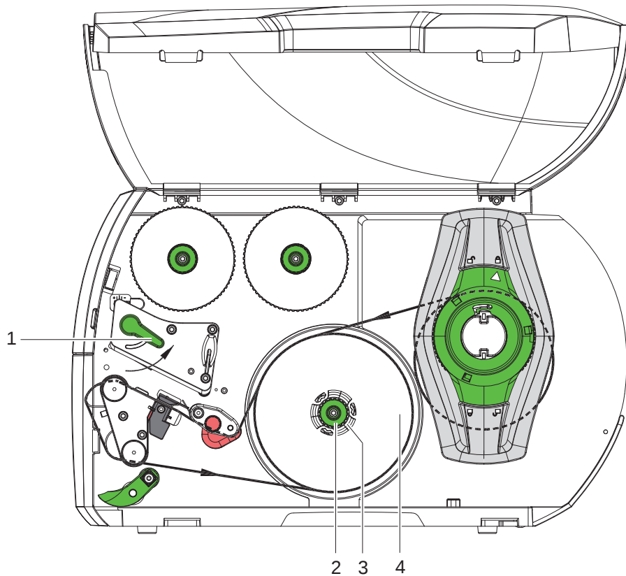
Bild 15 Aufgewickelte Rolle entnehmen
