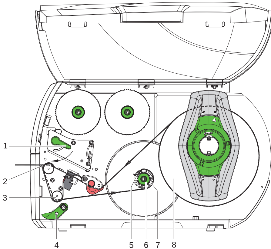
Bild 16 Führung des Materials im Spendemodus
