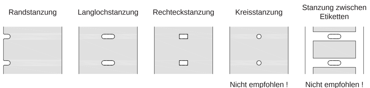
Bild 30 Beispiele für Stanzungen
