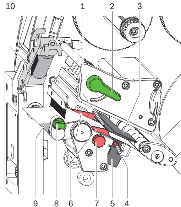
Geräte mit zentrierter Materialführung
