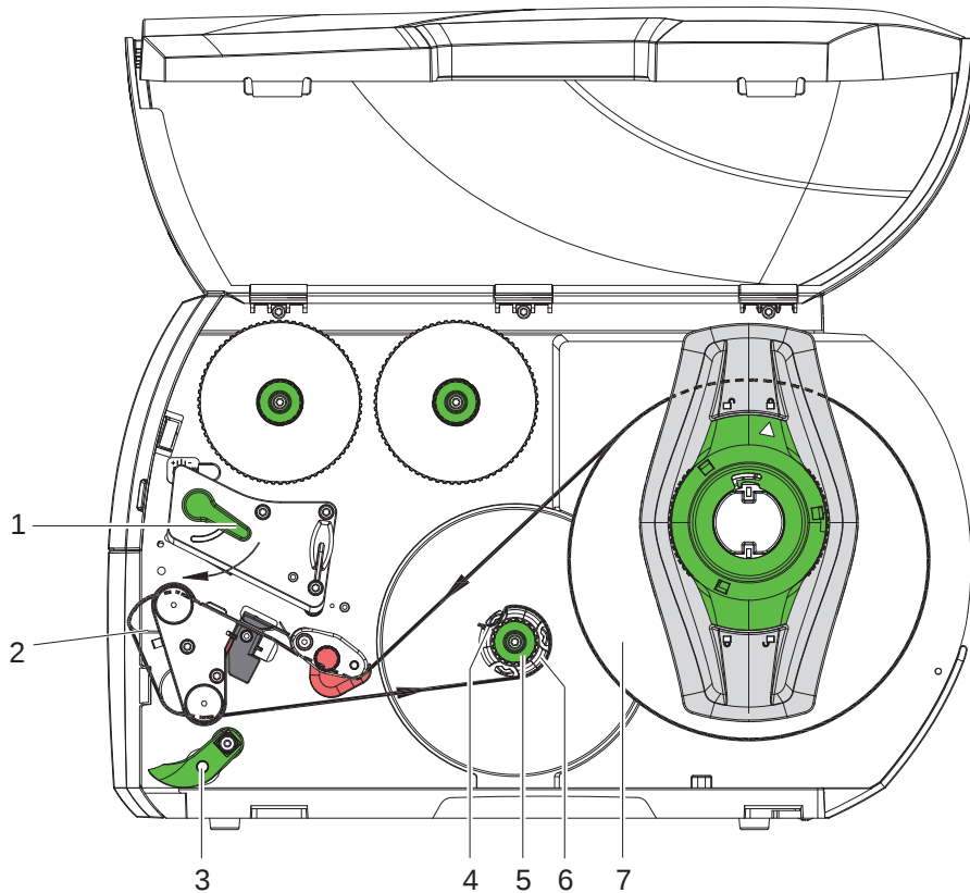
Bild 14 Führung der Etiketten im Aufwickelmodus
