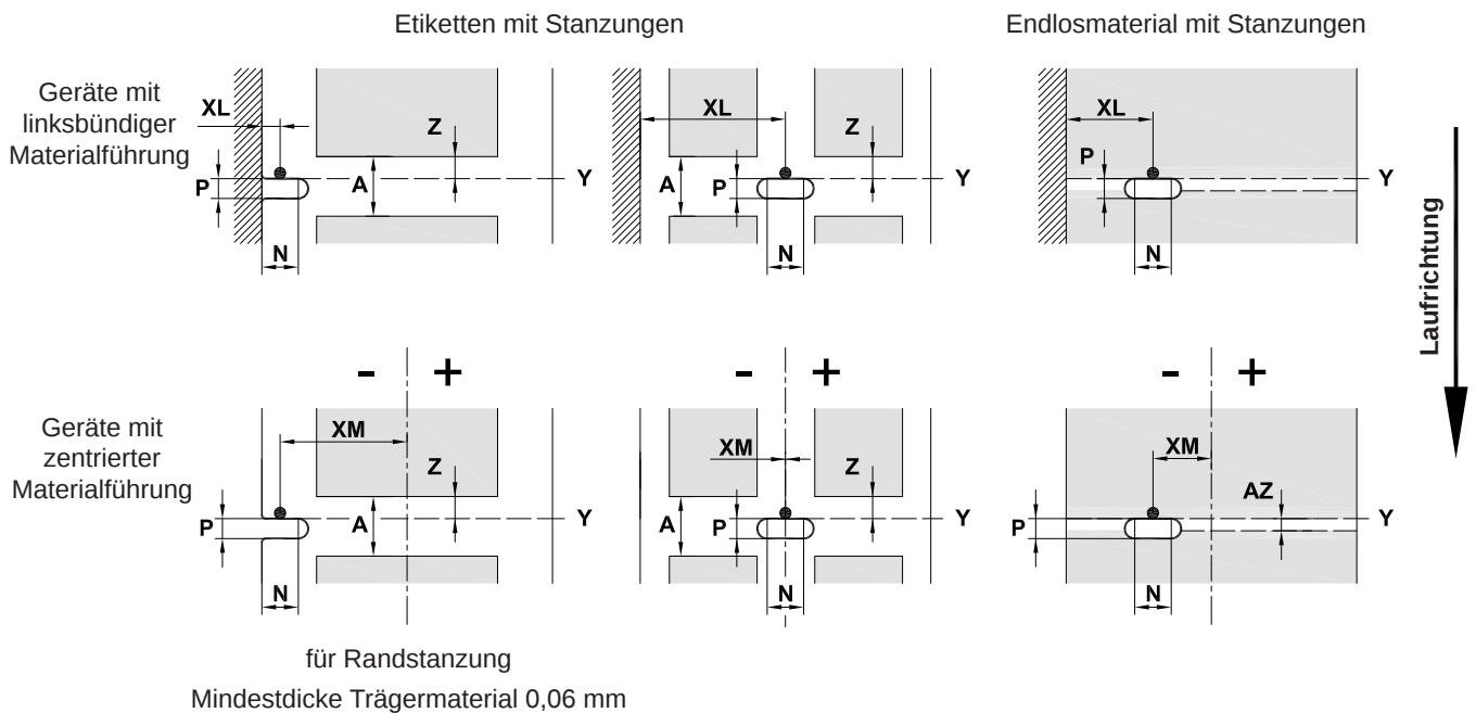
Bild 29 Maße für Stanzungen
