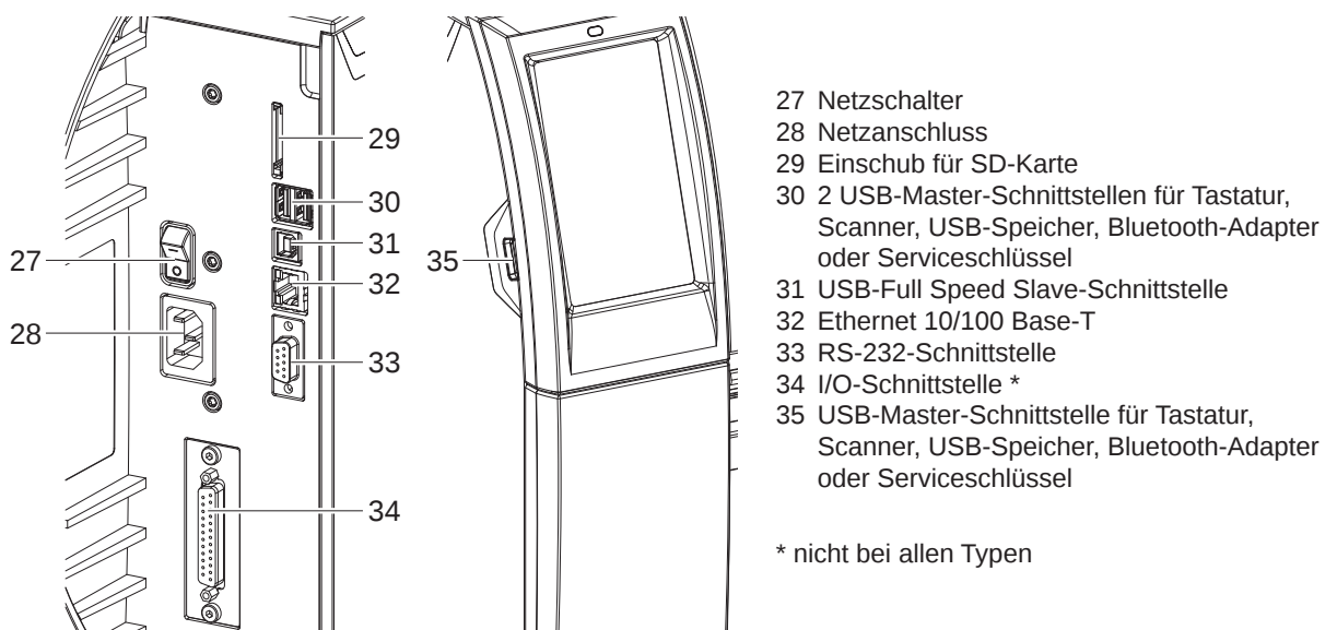
Bild 5 Anschlüsse
