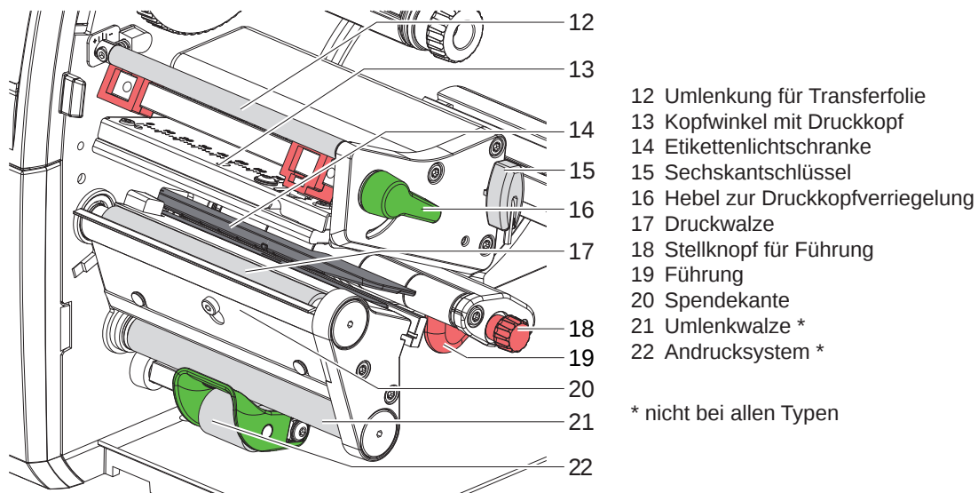
Bild 2 Druckbaugruppe - Geräte mit linksbündiger Materialführung
