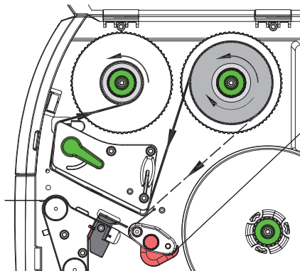
Bild 22 Transferfolienlauf
