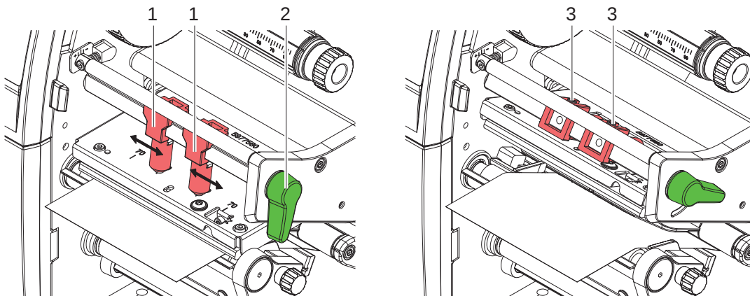
Bild 19 Kopfandrucksystem einstellen - Geräte mit zentrierter Materialführung
