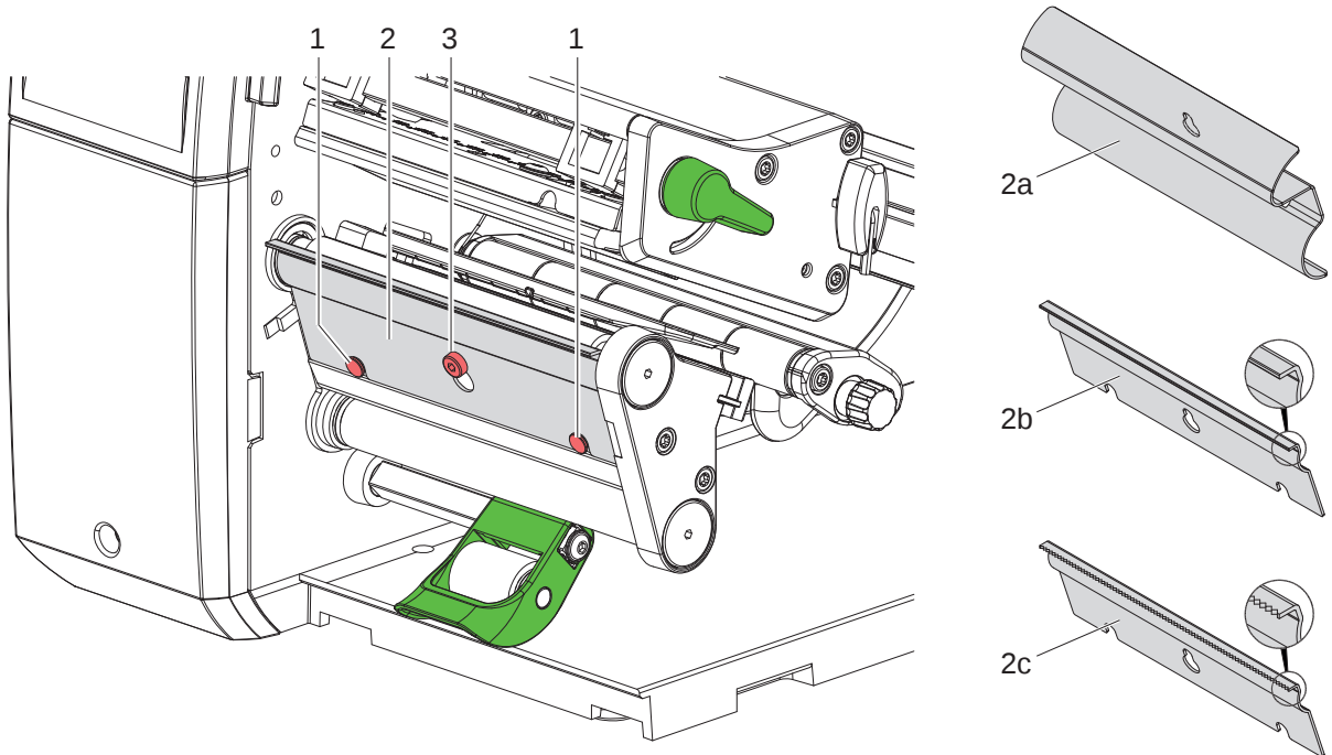
Bild 20 Umlenblech, Spende- oder Abreißkante ab- und anbauen
