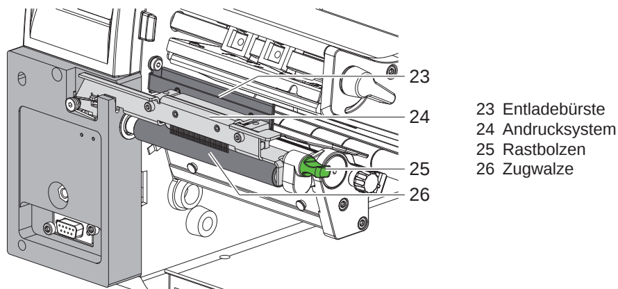
Bild 4 Separator an SQUIX MT
