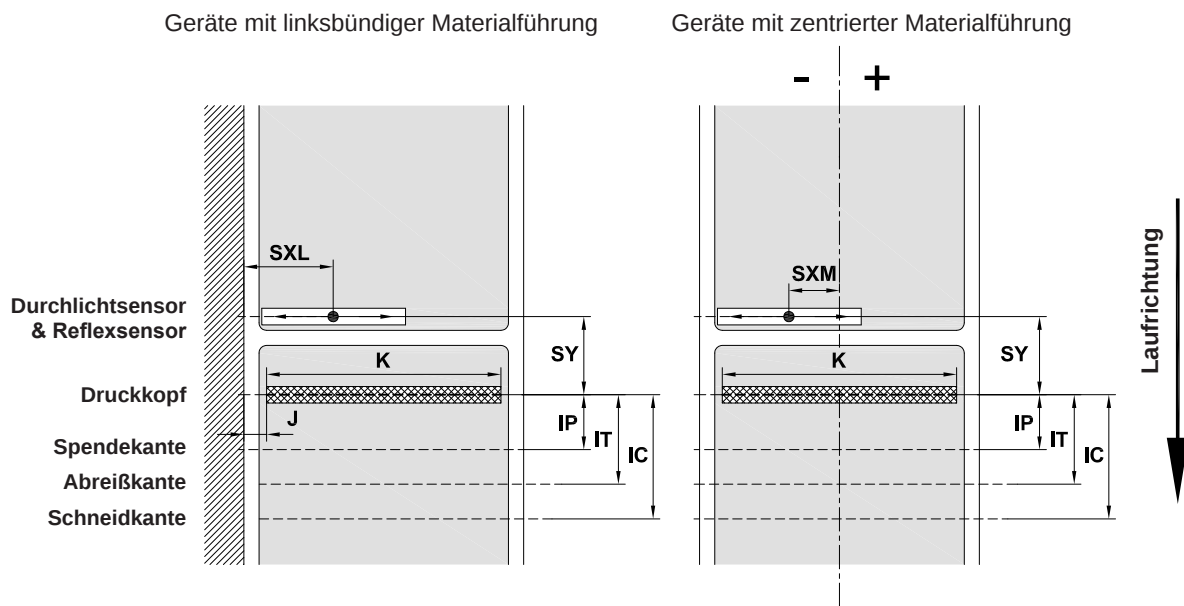
Bild 27 Gerätemaße
