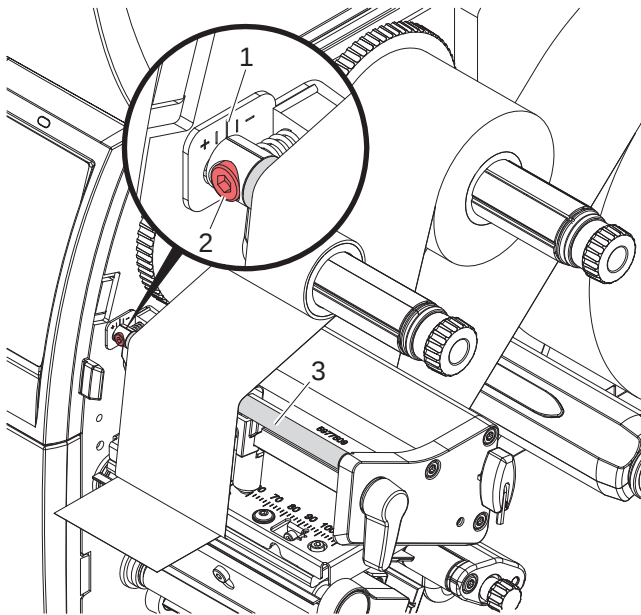
Bild 23 Transferfolienlauf einstellen
