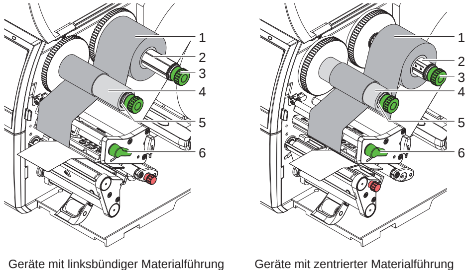
Bild 21 Transferfolie einlegen
