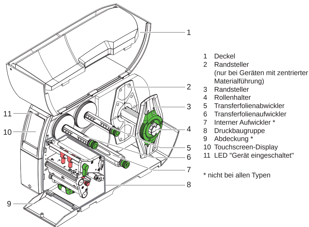
Bild 1 Übersicht
