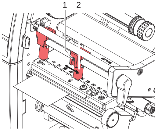
Bild 18 Kopfandrucksystem einstellen - Geräte mit linksbündiger Materialführung
