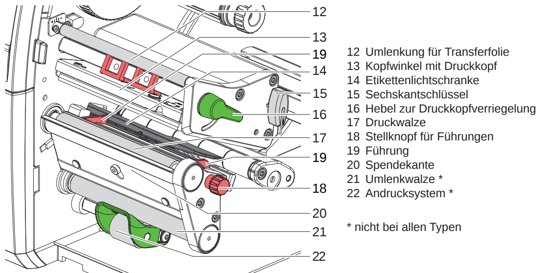
Bild 3 Druckbaugruppe - Geräte mit zentrierter Materialführung
