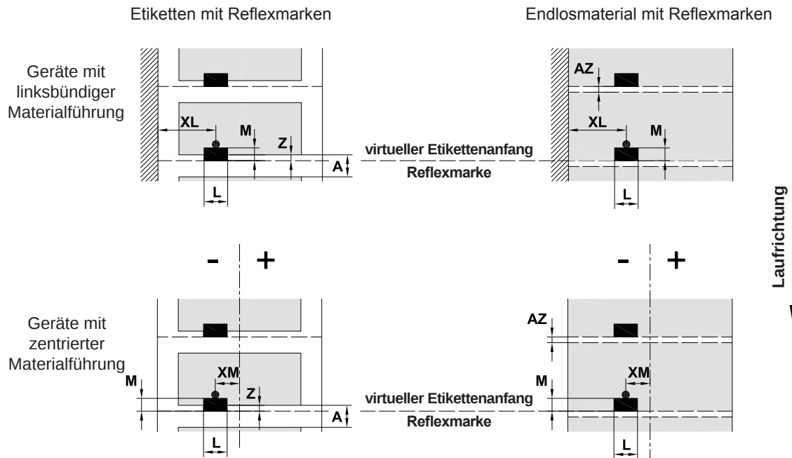
Bild 28 Maße für Reflexmarken
