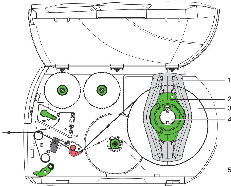
Bild 12 Rollenmaterial einlegen
