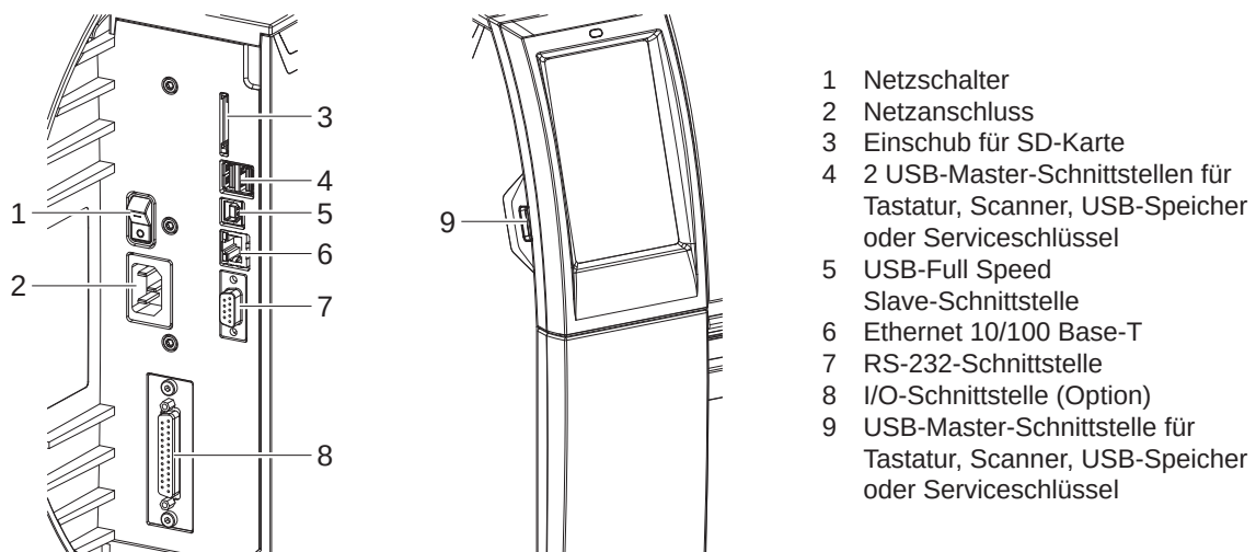
Bild 1 Anschlüsse
