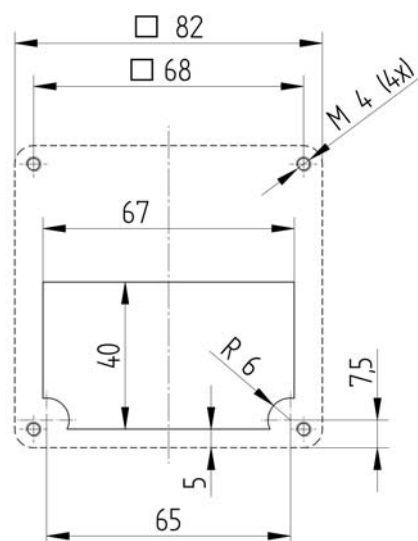
Montageausschnitt Panel cut-out
