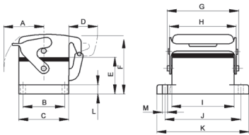
EPIC® HA/HB Base de superficie; palanca sencilla
