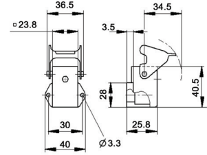
EPIC® HA 3/4 Base en ángulo; palanca sencilla
