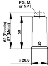
EPIC® HA 3/4 Tapa con entrada superior; pernos sencillos
