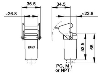
EPIC® HA 3/4 Tapa de cople de conexión; palanca sencilla
