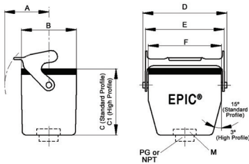
EPIC® HA/HB Tapa de cople de conexión; palanca sencilla
