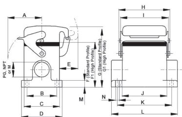
EPIC® HA/HB Base de superficie; palanca sencilla
