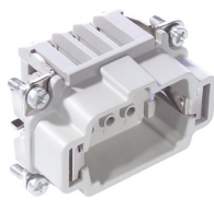
Terminación crimpada Contactos no incluidos
