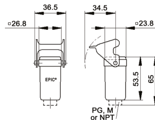
EPIC® HA 3/4 Tapa de cople de conexión; palanca sencilla
