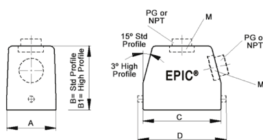
EPIC® HA/HB Tapa con entrada superior y lateral; pernos sencillos
