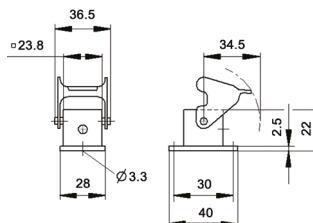
EPIC® HA 3/4 Base de panel; palanca sencilla
