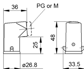
EPIC® HA 3/4 Tapa con entrada lateral pernos sencillos
