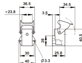
EPIC® HA 3/4 Base en ángulo; palanca sencilla
