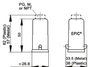
EPIC® HA 3/4 Tapa con entrada superior; pernos sencillos
