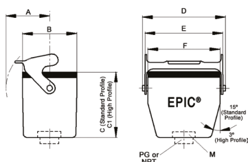
EPIC® HA/HB Tapa de cople de conexión; palanca sencilla
