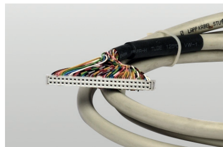
UNITRONIC® LiYY z płaskim złączem Zastosowanie: Panele sterownicze
