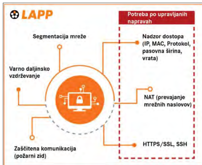
Slika 3: Varnost omrežja [1]
