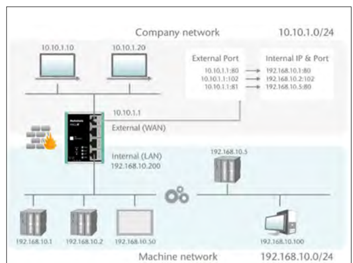
Slika 6: NAPT [2]
