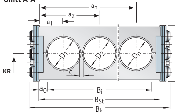
Snitt A-A
