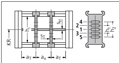
TS1, vertikal och genomgående horisontell avdelning.
