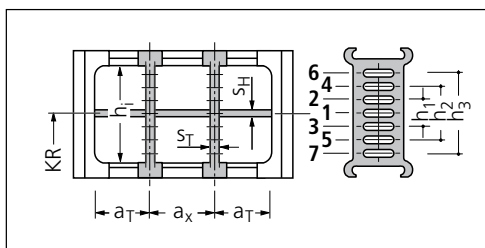
Vertikal och genomgående horisontell avdelning. Endast för S/SX 1250. Den horisontella avdelaren är i aluminium.
