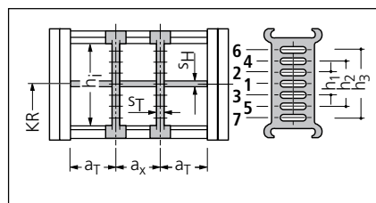
TS1, vertikal och genomgående horisontell avdelning.
