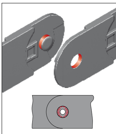
■ Kraftöverföring via sprintkoppling.
