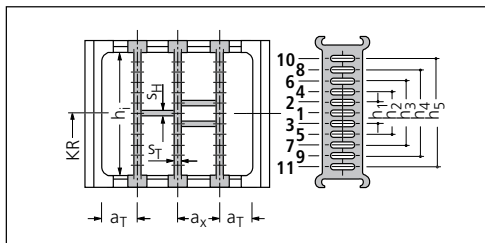
Vertikal och horisontell sektionerad avdelare. Den horisontella avdelaren är av plast och finns i flera bredder. Endast för S/SX 1800.
