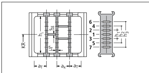
Vertikal och horisontell sektionerad avdelare. Den horisontella avdelaren är i aluminium. Endast för S/SX 1250.
