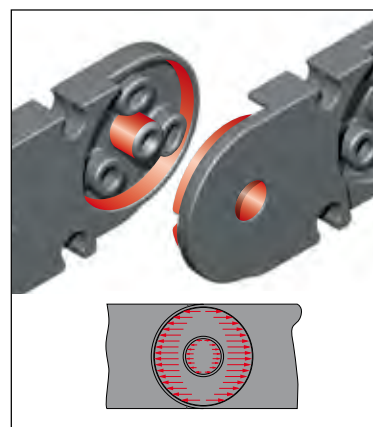
■ Kraftöverföring med "livsförlängande 2-skiveprincip".
