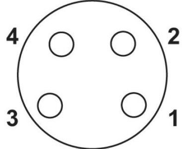
Polbild M8-Buchse, 4-polig, A-kodiert, Ansicht Buchsenseite
