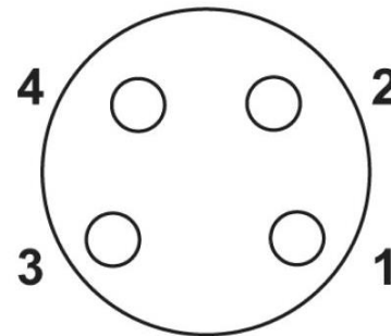
Schaltplan
