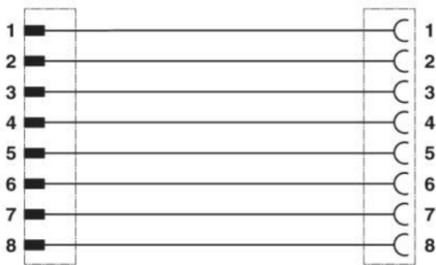
Kontaktbelegung des M12-Stecker und der M12-Buchse
