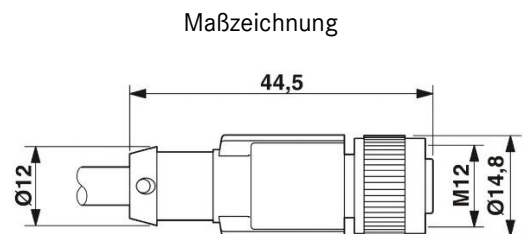
Buchse M12 x 1, gerade
