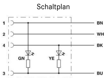
Kontaktbelegung der M12-Buchse mit LED
