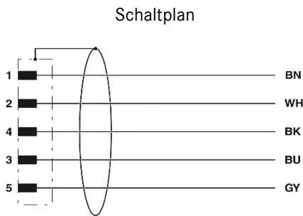
Kontaktbelegung des M12-Steckers
