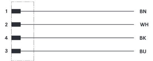
Kontaktbelegung des M12-Steckers
