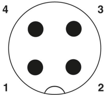
M12-Stecker, 4-polig, A-kodiert
