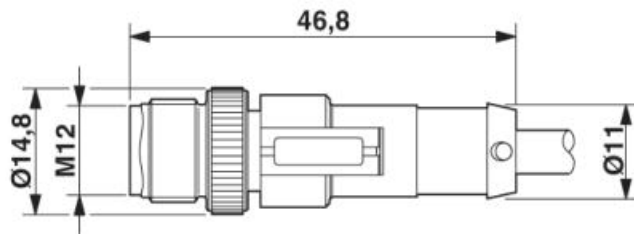
Stecker M12, gerade
