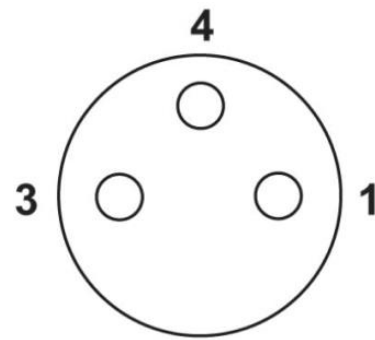
Pin assignment M8-jack, 3-pol, A-codiert
