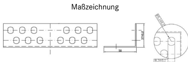
Verteilerplatte 12x ST/FC
