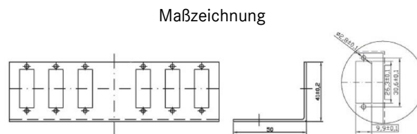
Verteilerplatte 6x SC-D/LC-Q
