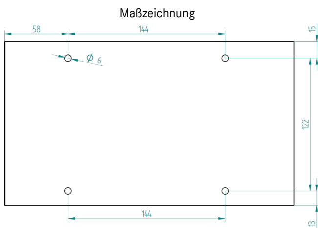
Wandmontage Bohrungen
